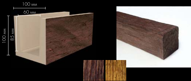
Балка 10-10
